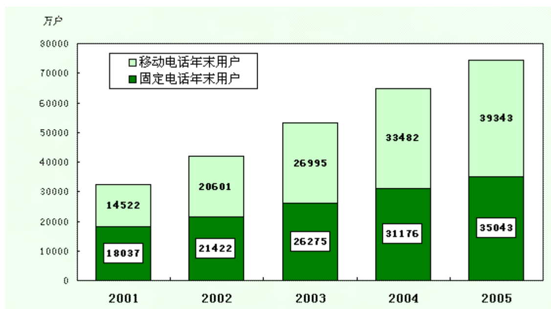
图 8 “十五”时期各年年末电话用户数
